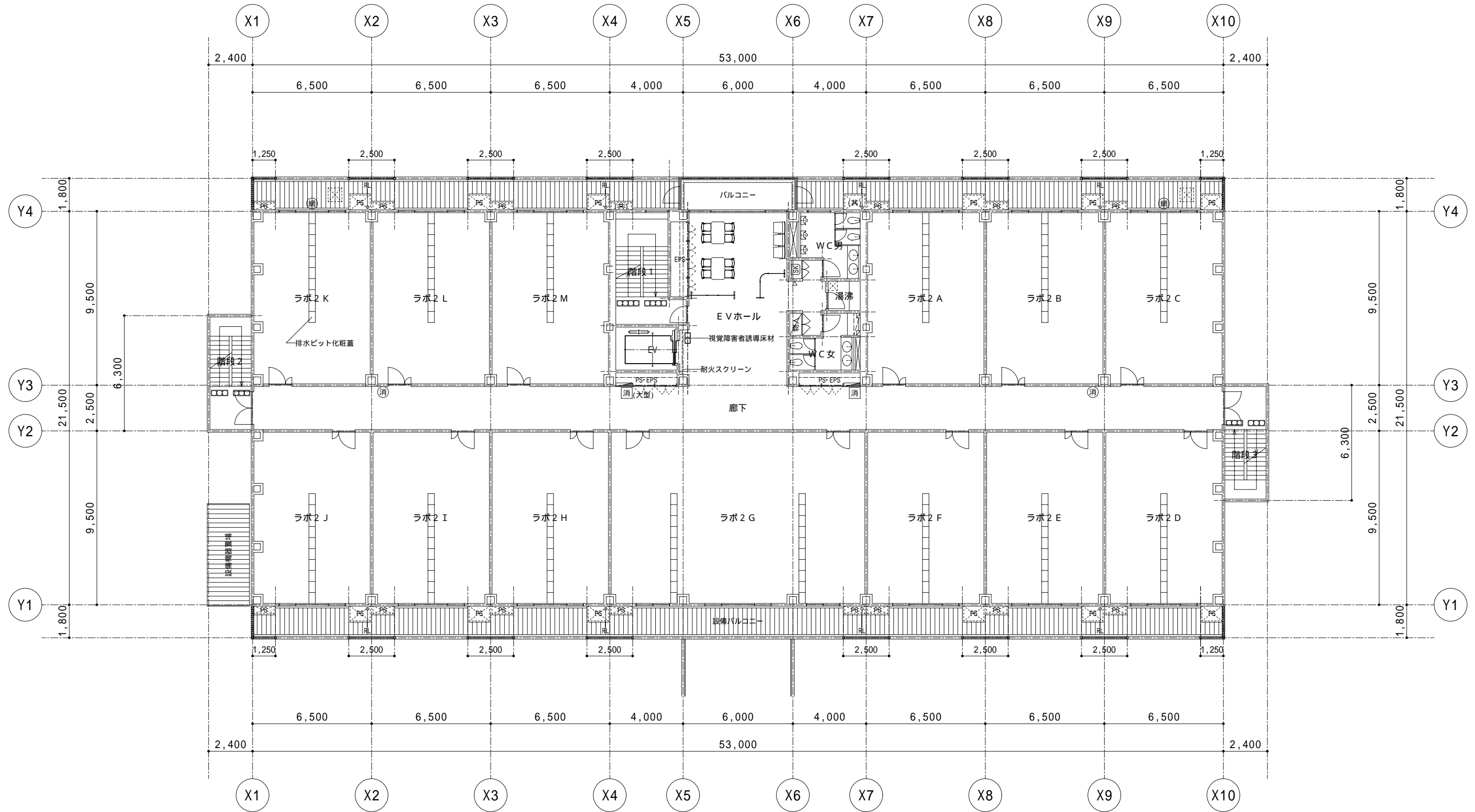
2階平面図
